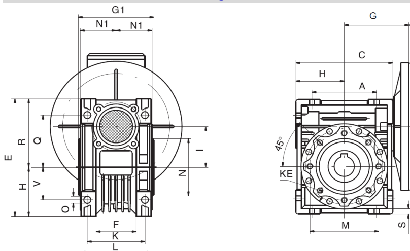
Input Flange
