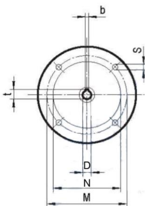
Input Flange
