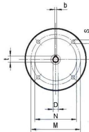
Input Flange
