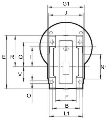
Input Flange
